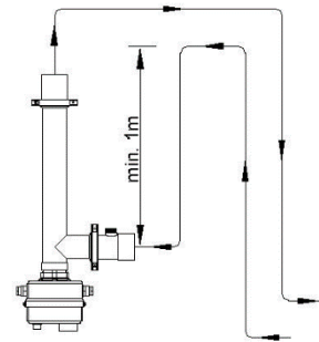
vertikaler Einbau
